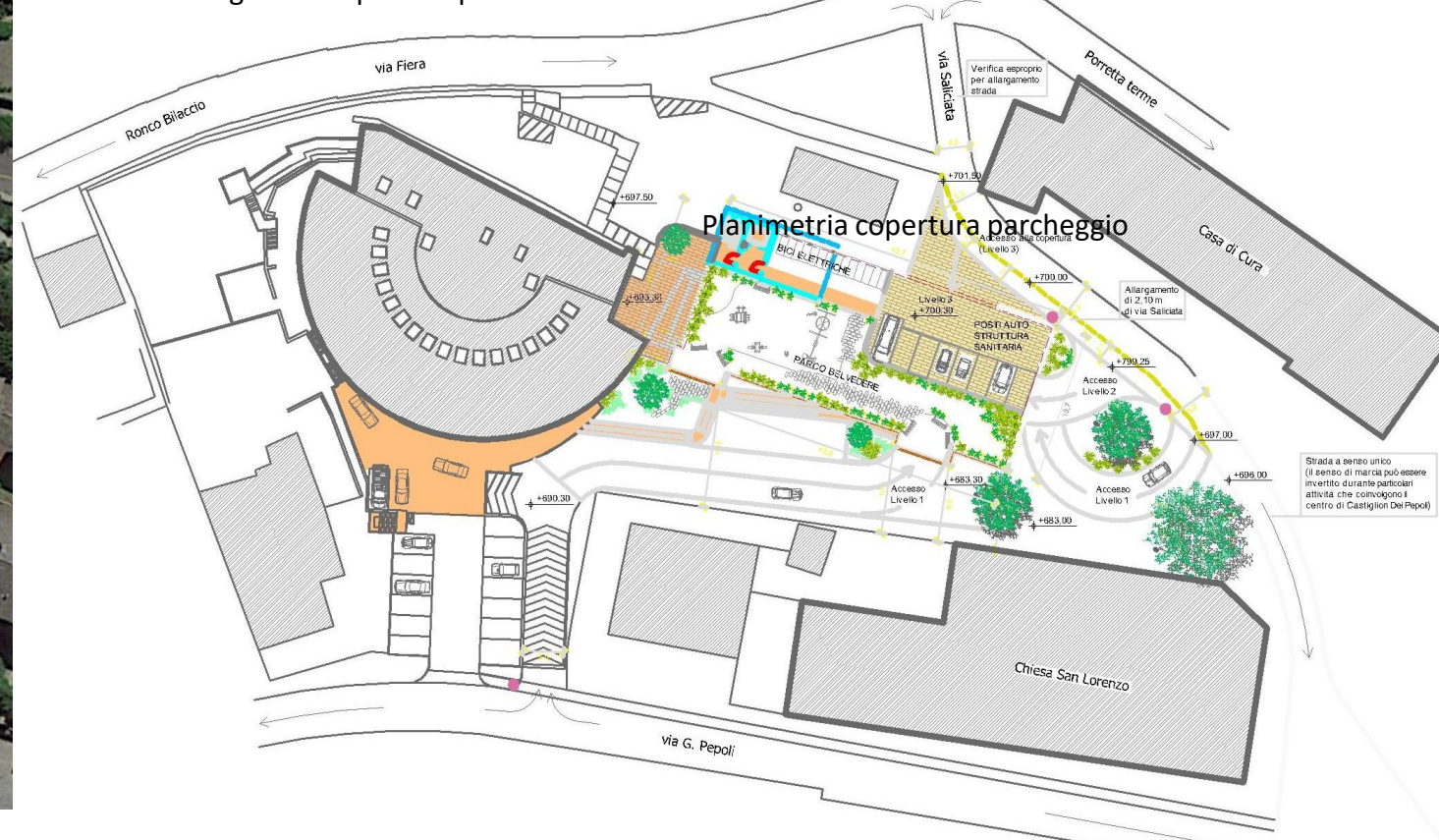
Planimetria generale quota copertura
